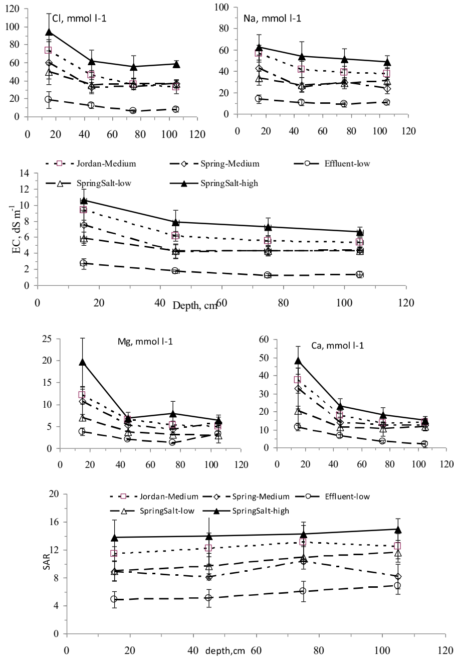
איור 1- השפעת טיפול ההשקיה על ריכוזי הכלוריד, נתרן, מוליכות חשמלית (EC), סידן והמגנזיום ועל ערכי ה-SAR כתלות בעומק הקרקע לפני תחילת הניסוי הנוכחי בשיקום הקרקע (אפריל 2008)
